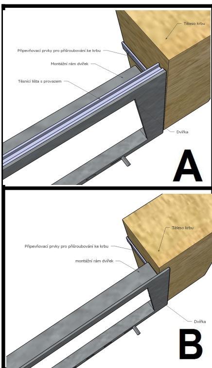
Dvířka dvoukřídlá
